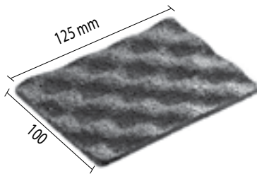
Vibro-Profi mat
